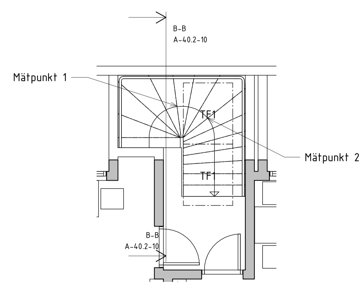
DETALJ TRAPPA
